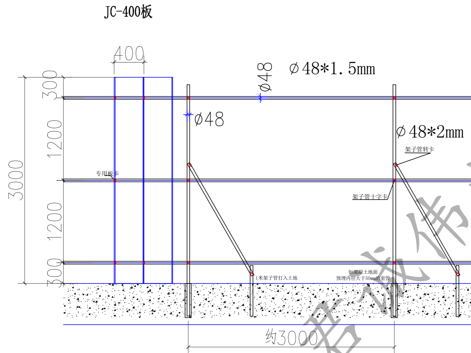
无基础安装方案 土地及混凝土安装
